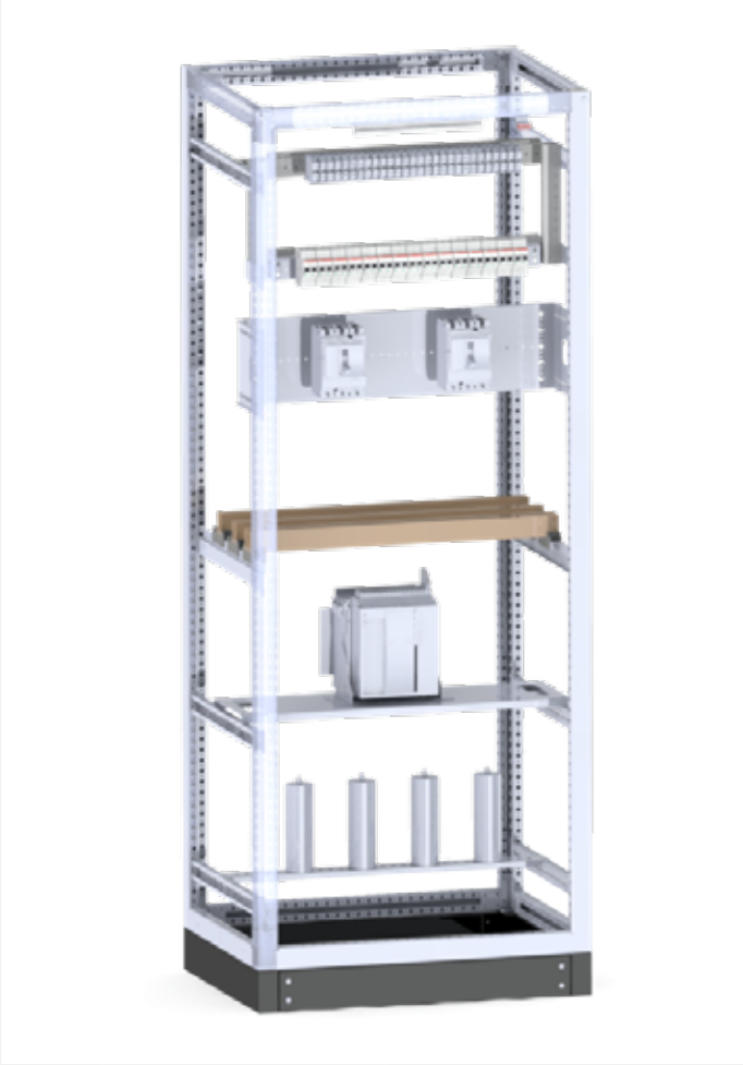
İç parça sistemi Internal part system
