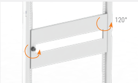
Menteşeli perde sacı, bütün pano serilerinde ortak kullanım Hinged cover plate, common use in all series
