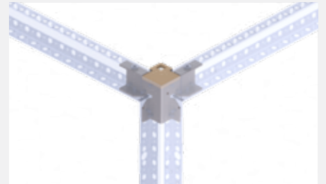
Profili mükemmel saran köşe birleşim sistemi Corner connection that perfectly surrounds profile
