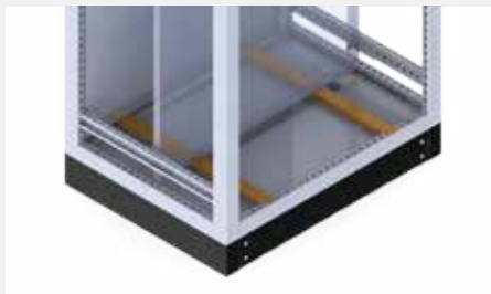
Taban sacı taşıma kızakları Base plate carrier slides
